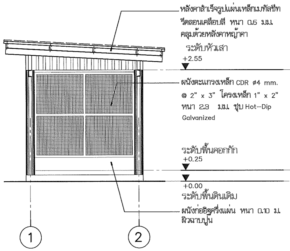
รูปด้าน 1 1:50
