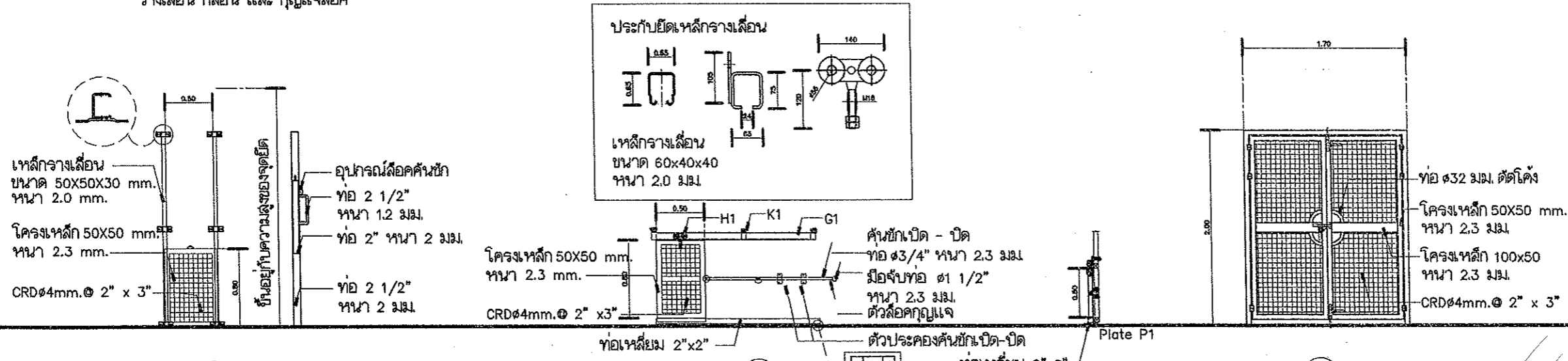
D4 ประตูบานยก โครงเหล็กประตู 50 X 50 mm. หน้า 2.3 mm. พร้อมอุปกรณ์ระบบยก ลลิ่งเชือกถักโพลีเอสเตอร์ 6 มม. รางเลื่อน กลอน และ กุญแจล็อก
