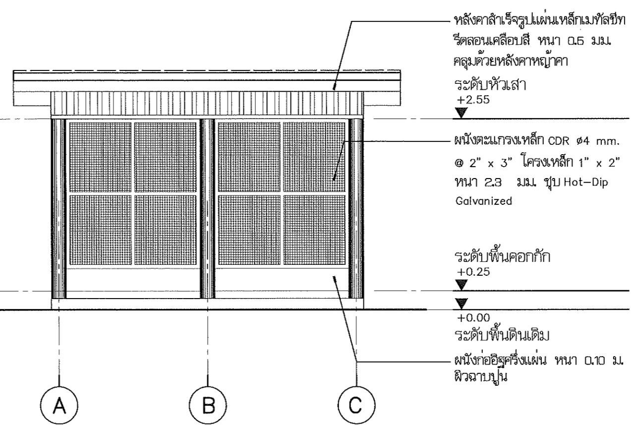
รูปด้าน 2 1:50
