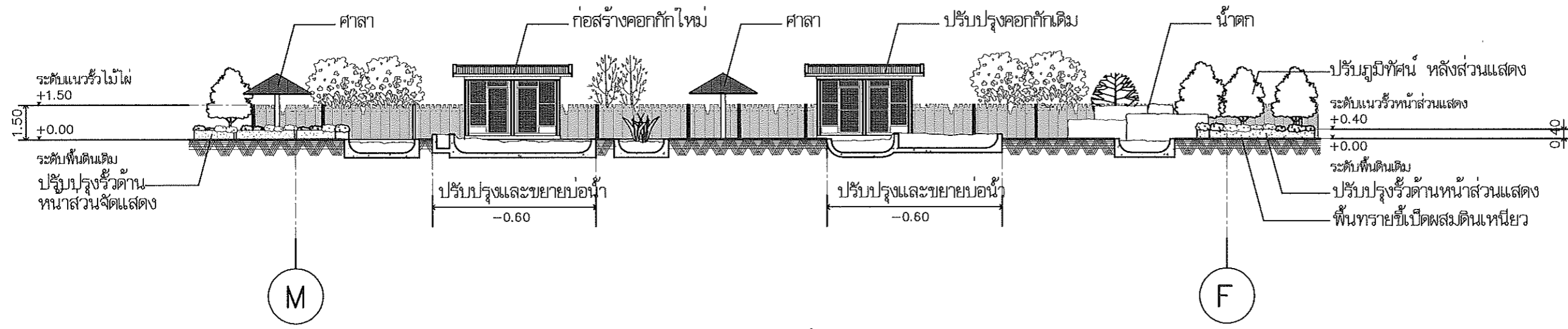
รูปตัด A-A 1:200
