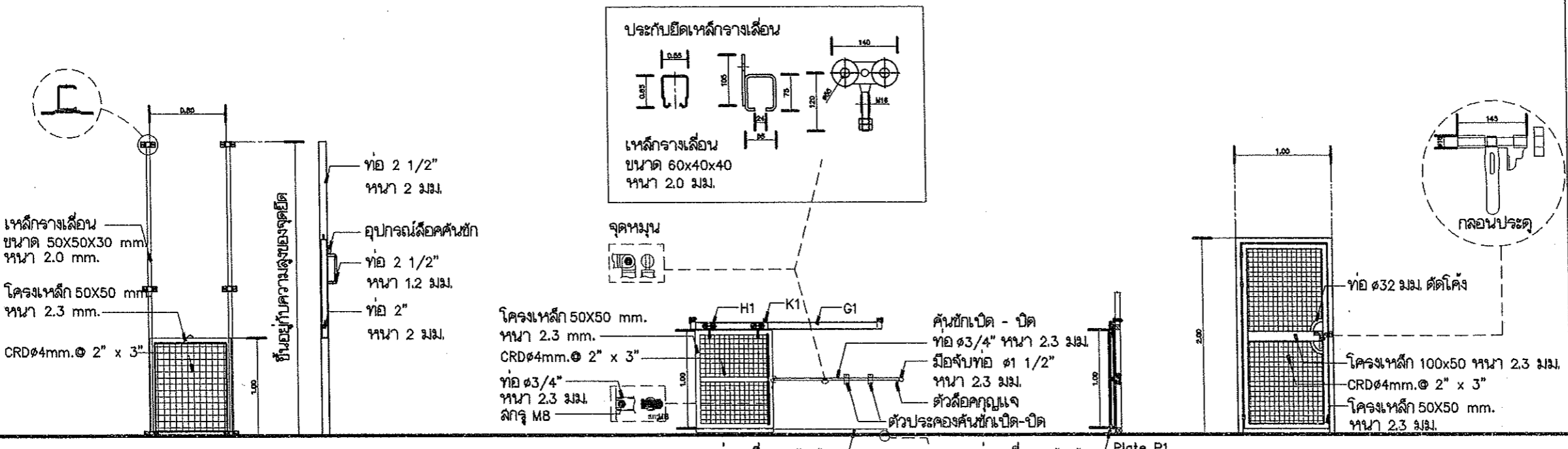
D1 ประตูบานยก โครงเหล็กประตู 50 X 50 mm. หน้า 2.3 mm. พร้อมอุปกรณ์ระบบยก ลลิ่งเชือกถักโพลีเอสเตอร์ 6 มม. รางเลื่อน กลอน และ กุญแจล็อก
