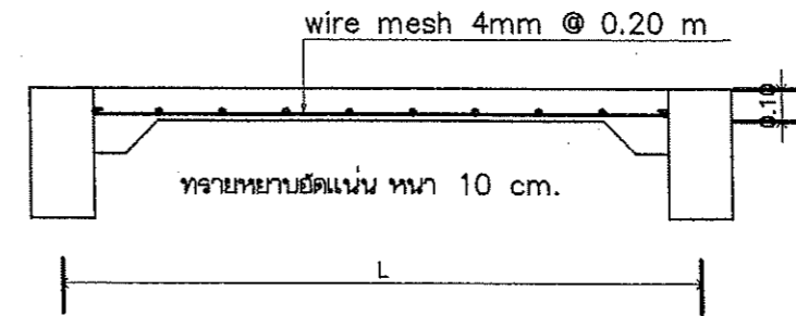
(GS) แบบขยายพื้น
