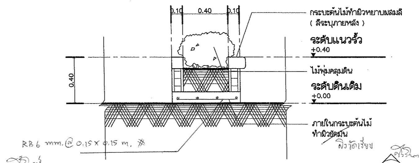
รูปตัด
