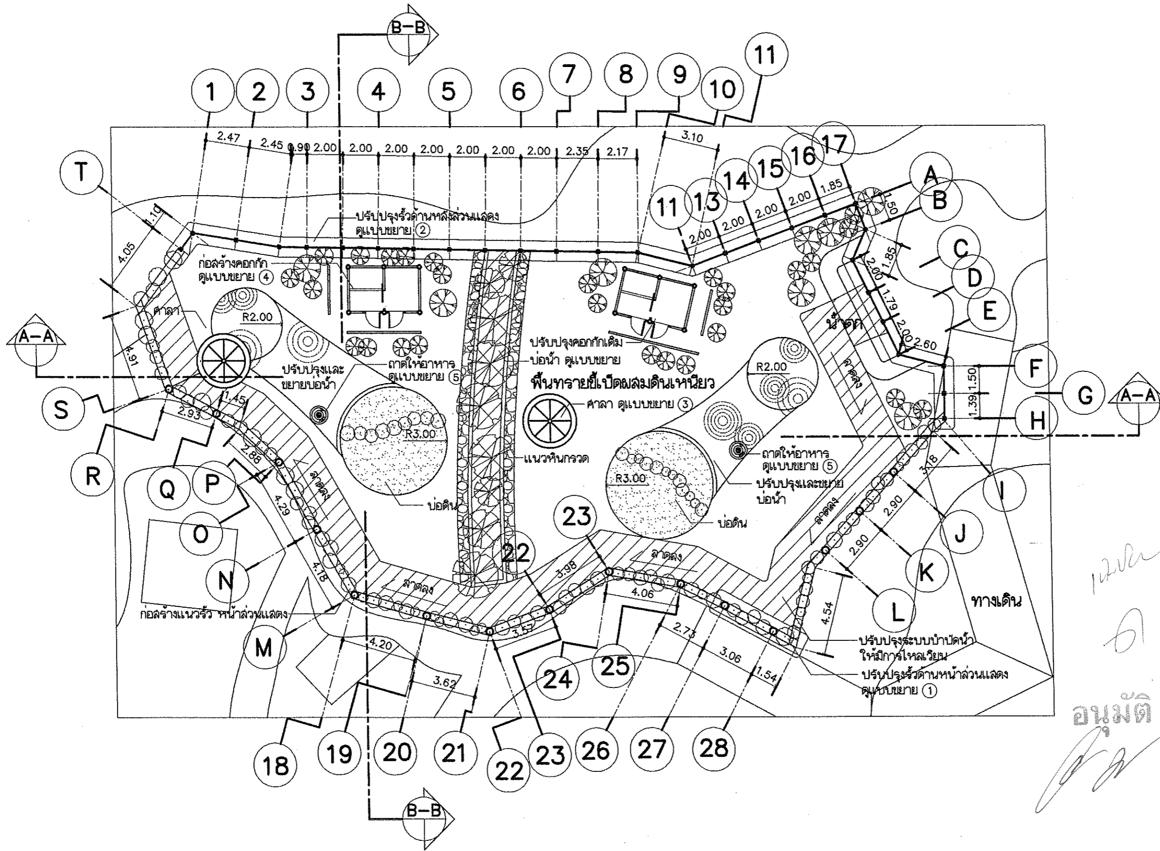
แบบผังรวมส่วนจัดแสดง ( ส่วนจัดแสดงพามิงโก้ )
