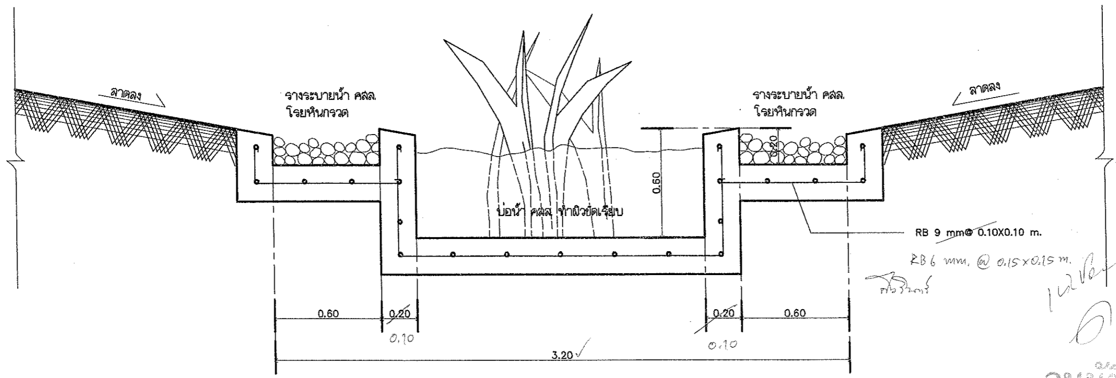
รูปตัด
