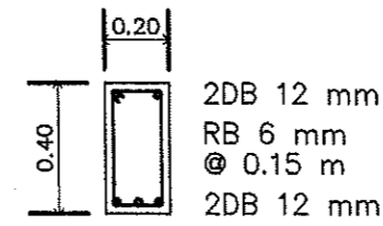
(GB1) แบบขยายคาน
