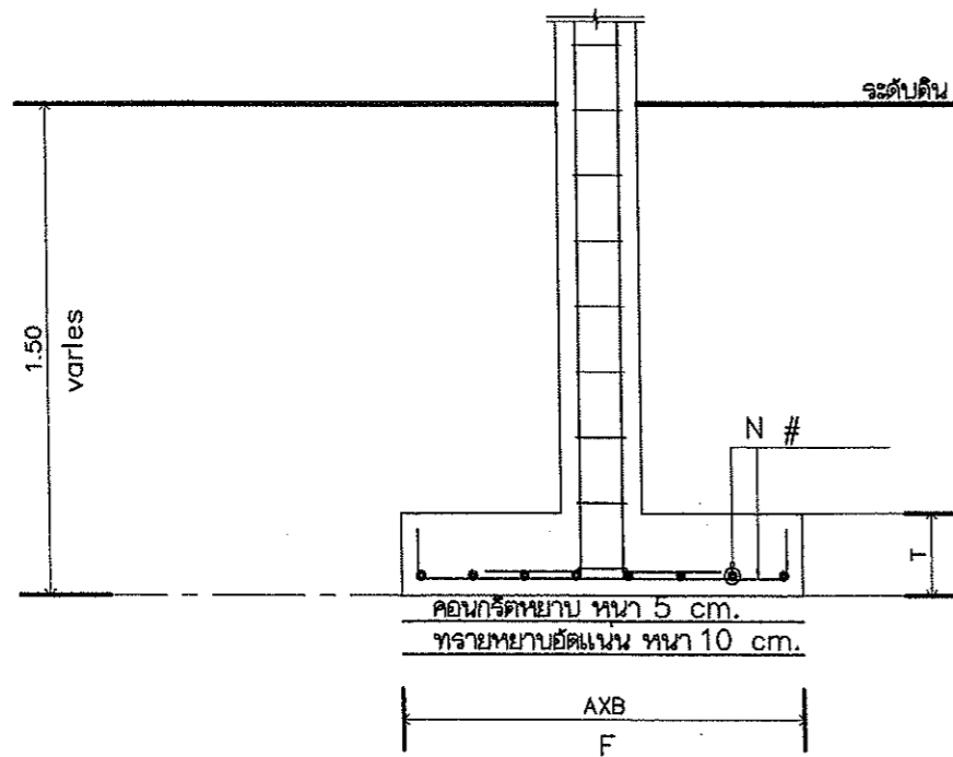
แบบขยายฐานราก
