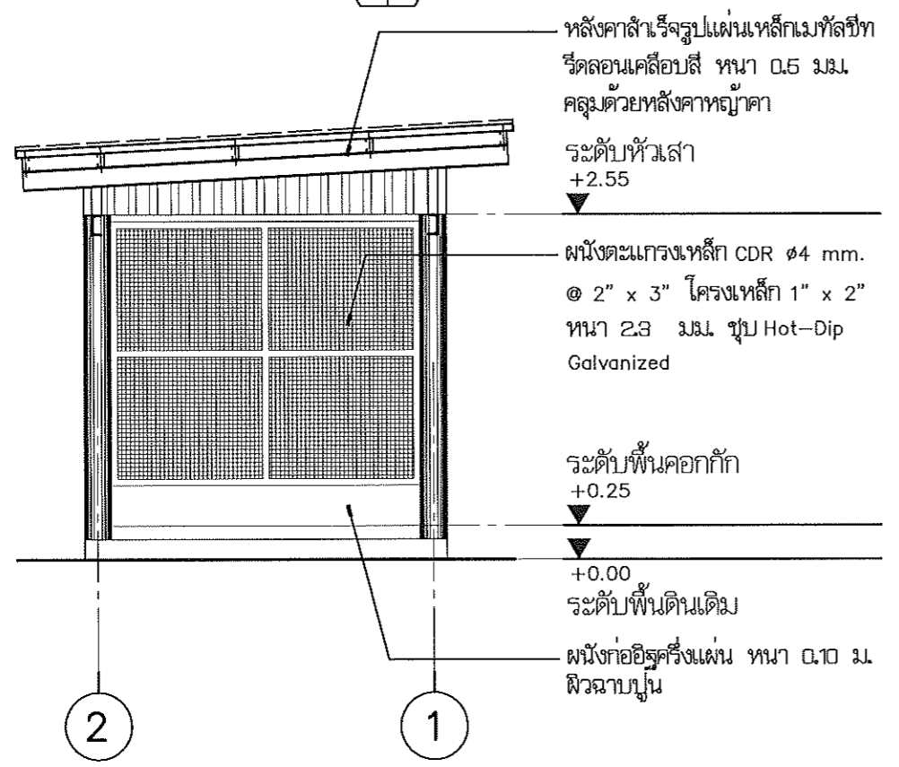
รูปด้าน 3 1:50
