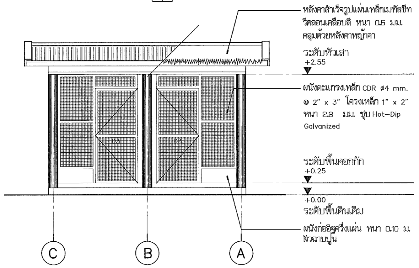
รูปด้าน 4 1:50
